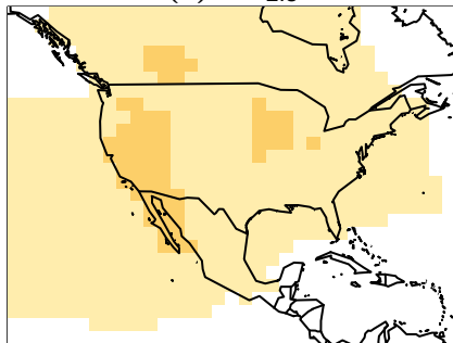
(d) Ozone
